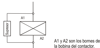
Esquema de conexión de Supresores en cargas con activación directa
