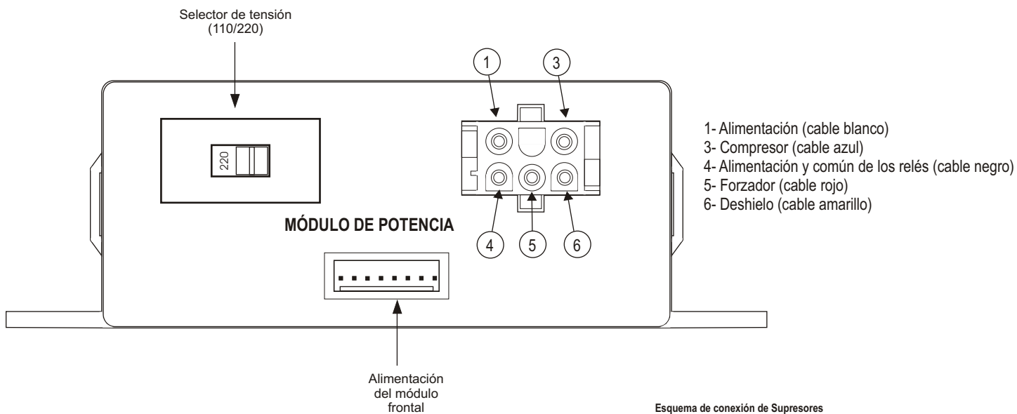
Esquema de conexión de Supresores en contactores
