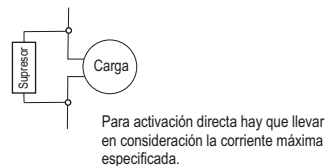
Esquema de conexión de Supresores en cargas con activación directa
